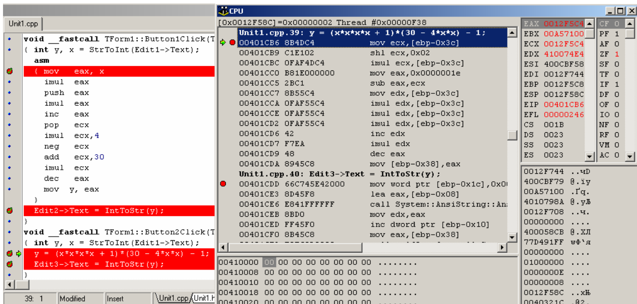
Рис. 1.2. Вигляд вікна дизасемблера для прикладу 1.2
