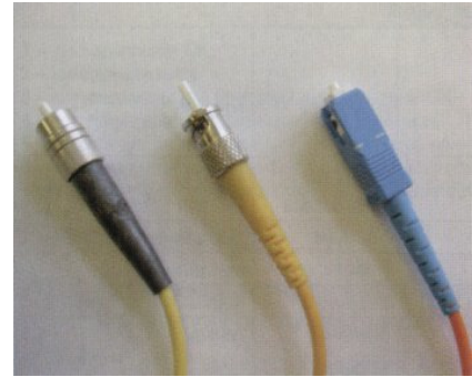
Рисунок 4.5 – Оптичні шнури, армовані з'єднувачами FC, SC, ST
