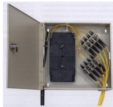
Рисунок 4.2 – Оптичне кросове обладнання шафного типу
