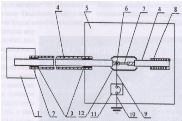
Рисунок 4.8 – Схема введення ОК в приміщення вузла зв'язку
