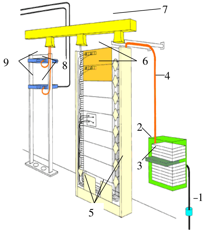
Рисунок 4.9 – Схема організації оптичного кросу
