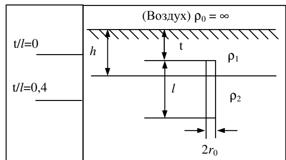
Рисунок 2.6 – График значений действующего удельного сопротивления грунта для трубчатых заземлителей:
