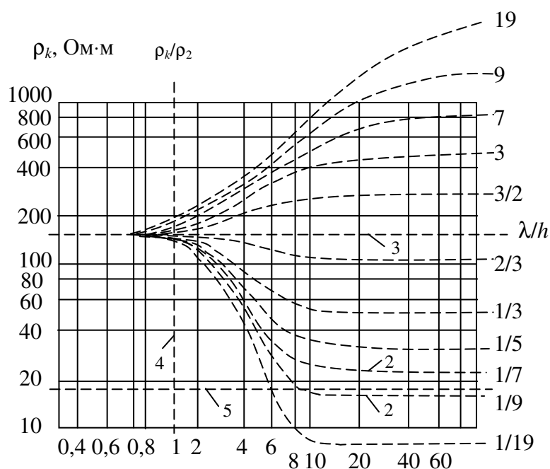
Рисунок 2.4 – Определение параметров грунта по кривым ВЭЗ с помощью палеток для двухслойной электрической структуры: 1 – кривая ВЭЗ, 2 – палетки, 3 – ось абсцис, 4 – ось ординат палеток, 5 – асимптота
