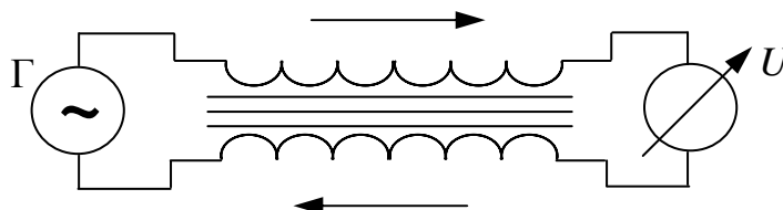
Рисунок 2.11 – Схема вимірювання втрат, які вносить запираюча котушка в коло сигналу
