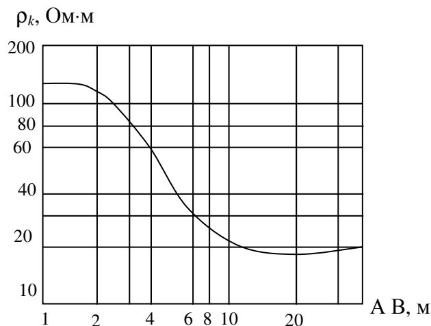
Рисунок 2.3 – Крива ВЕЗ
