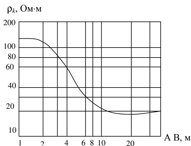
Рисунок 2.3 – Кривая ВЭЗ
