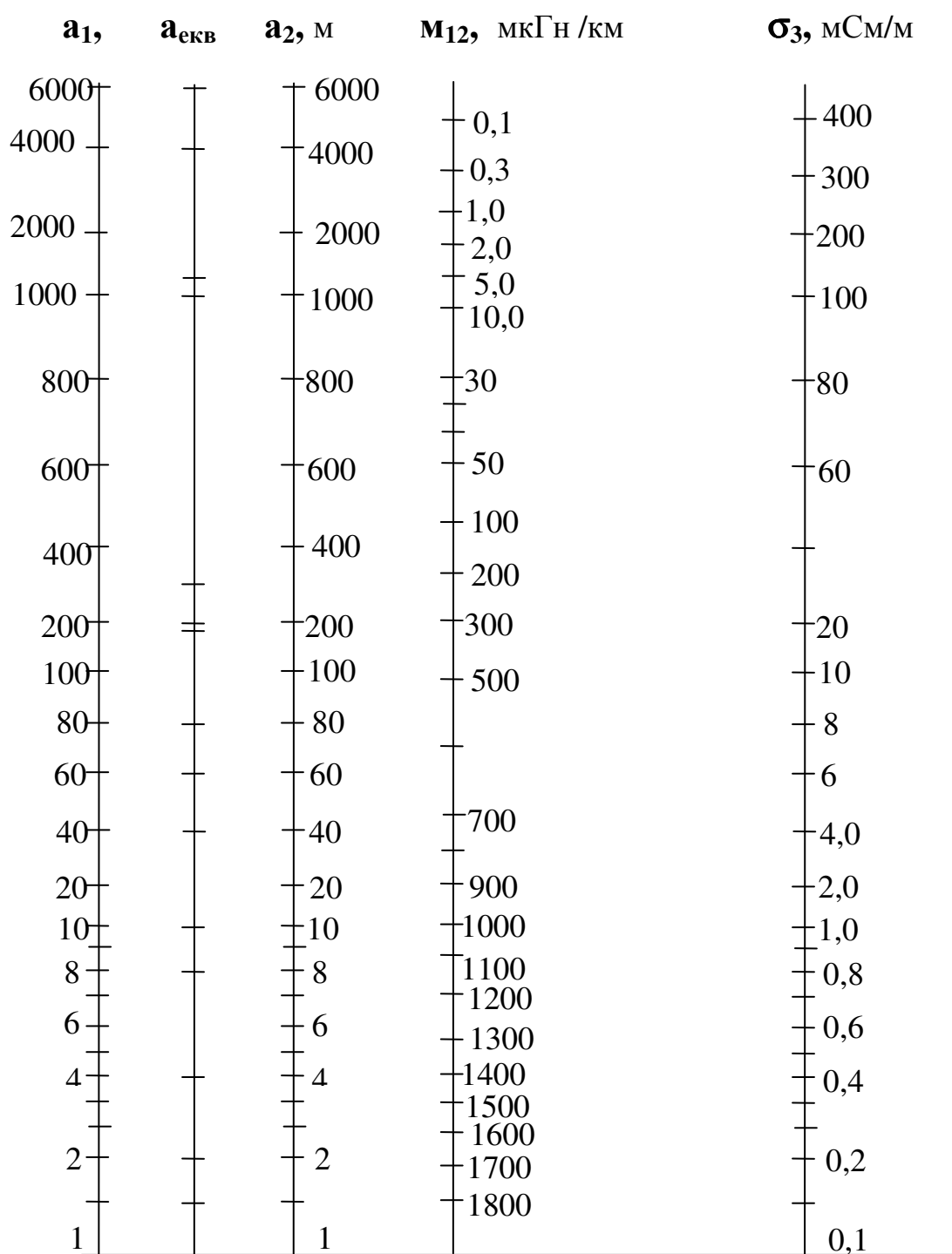
Рисунок 2.2 – Номограмма Михайлова
