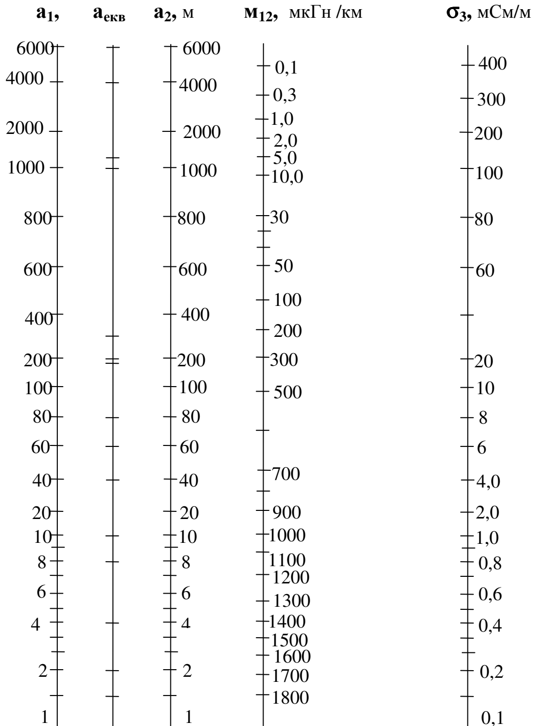
Рисунок 2.2 – Номограмма Михайлова
