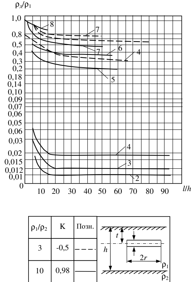
Рисунок 2.8 – Графік значень діючого питомого опору ґрунту для горизонтальних заземлювачів при різних відношеннях t/h и k<0 : 2 – t/h \geq 1,5 ; 3 – t/h = 1,1 ; 4 – t/h = 1,0 ; 5 – t/h = 0,9 ; 6 – t/h = 0,8 ; 7 – t/h = 0,4 ; 8 – t/h = 0,05 .
