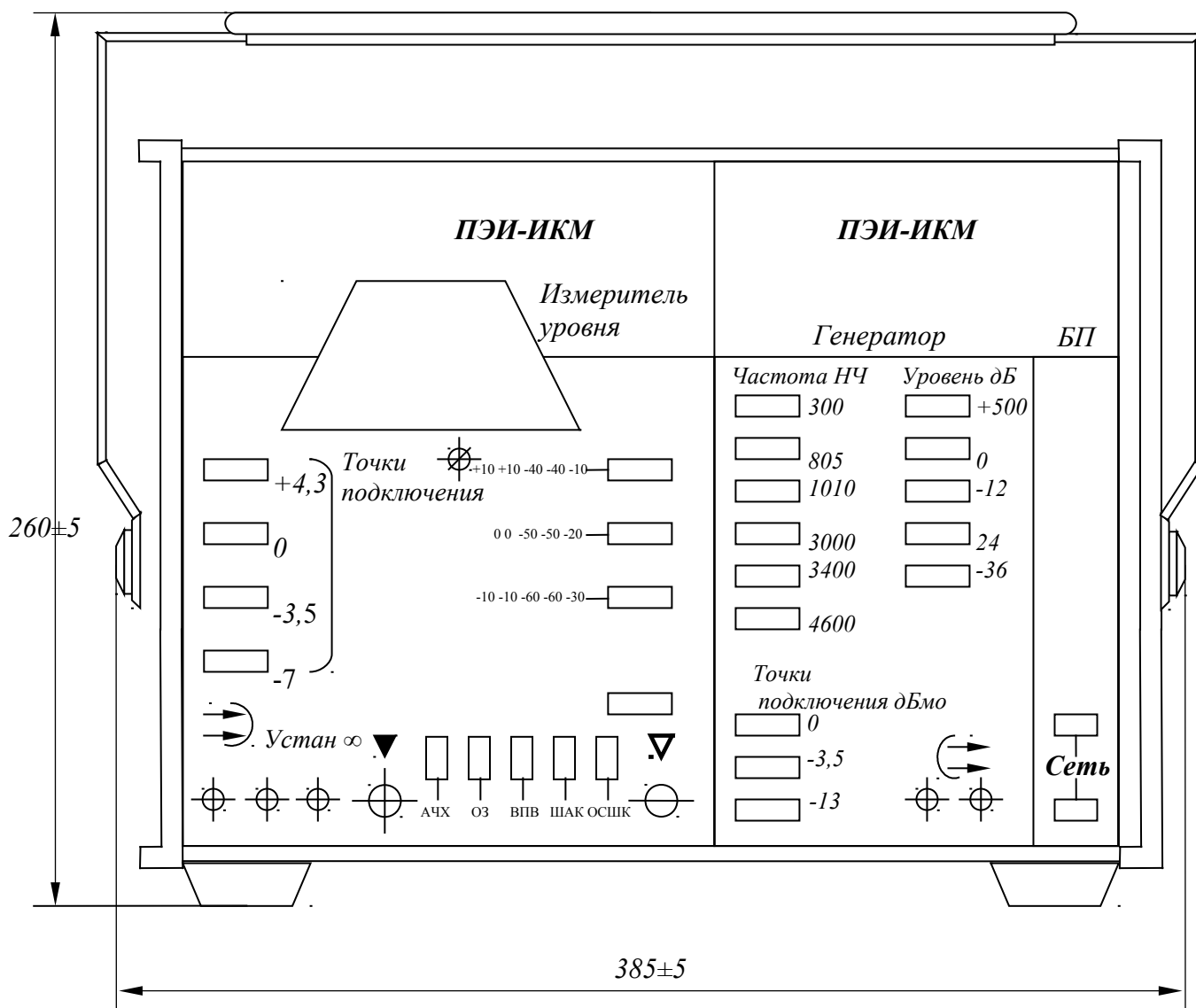
Рис. 6.1. Внешний вид фасадной панели прибора ПЭИ ИКМ
