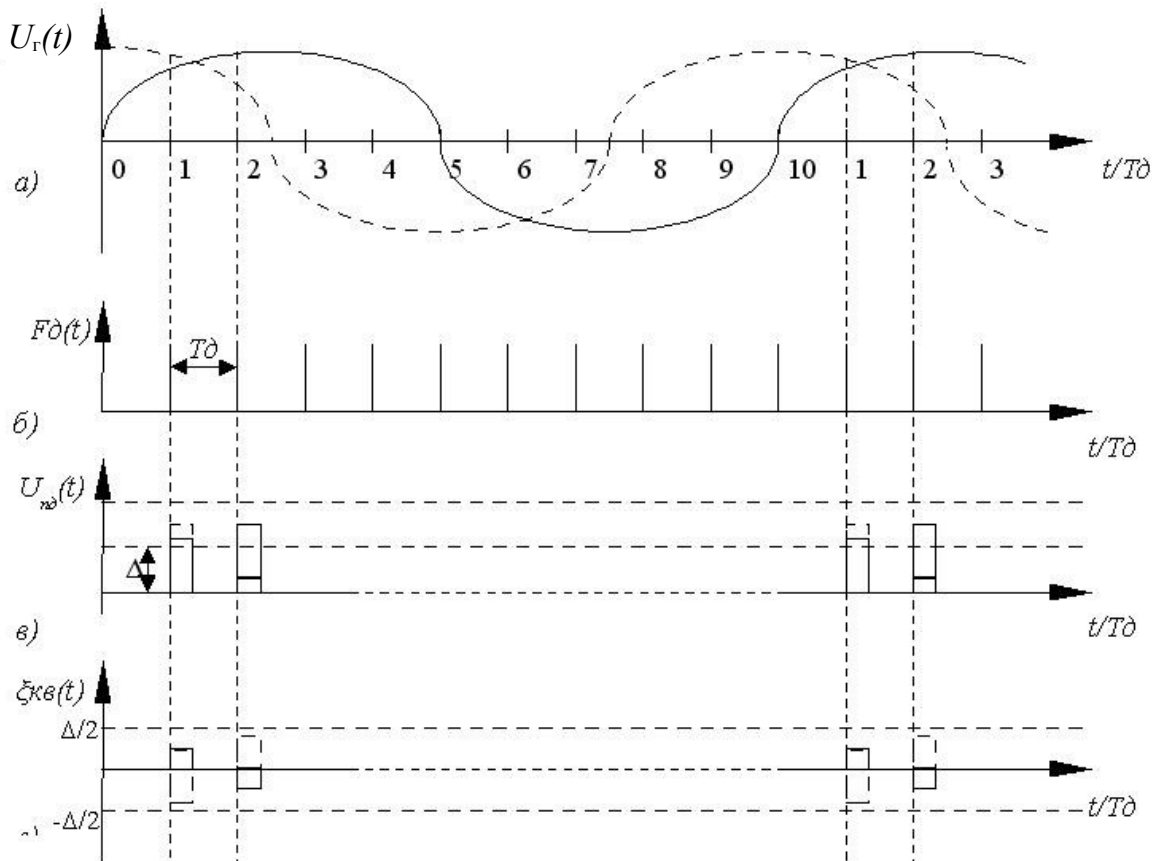
Рис. 2.1 Квантування і дискретизація гармонічного сигналу f_{\text{в}} = 800 Гц з різною початковою фазою
