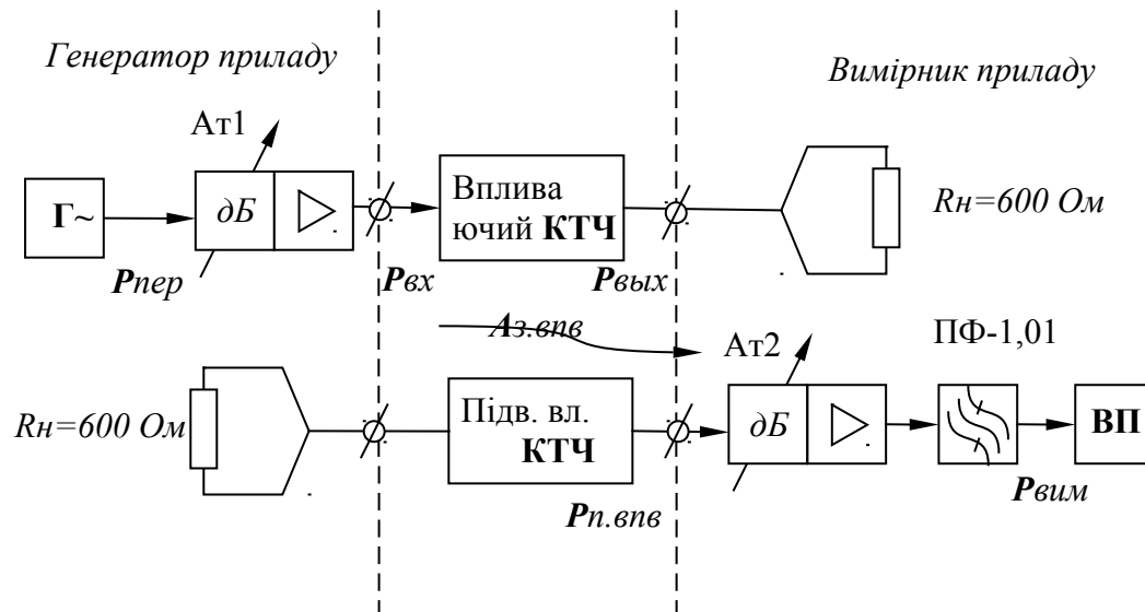
Рис. 2.10 – Схема вимірювання захищеності від виразних переходів впливу між КТЧ
