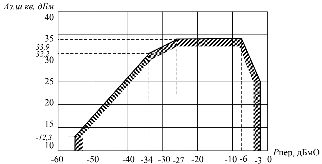
Рис. 2.7 – Шаблон захищеності від шумів квантування в КТЧ при вимірюванні псевдовипадковим сигналом
