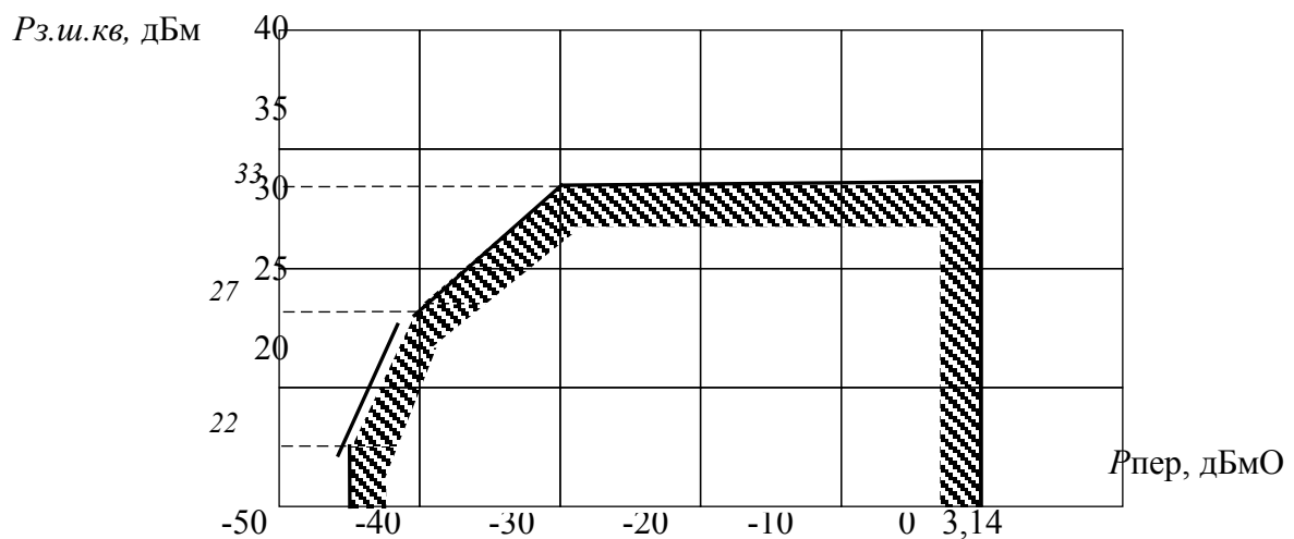
Рис. 2.8 – Шаблон захищеності від шумів квантування в каналі ТЧ при вимірюванні гармонічним сигналом = 1010 Гц
