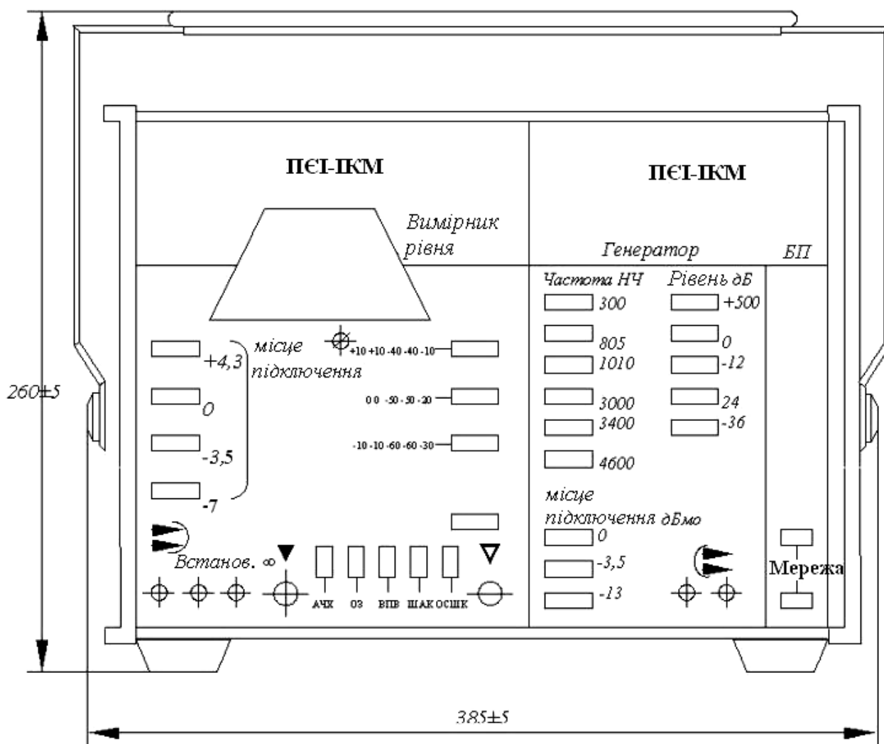
Рис. 6.1. Зовнішній вигляд лицьової панелі приладу ПЕІ- ІКМ.
