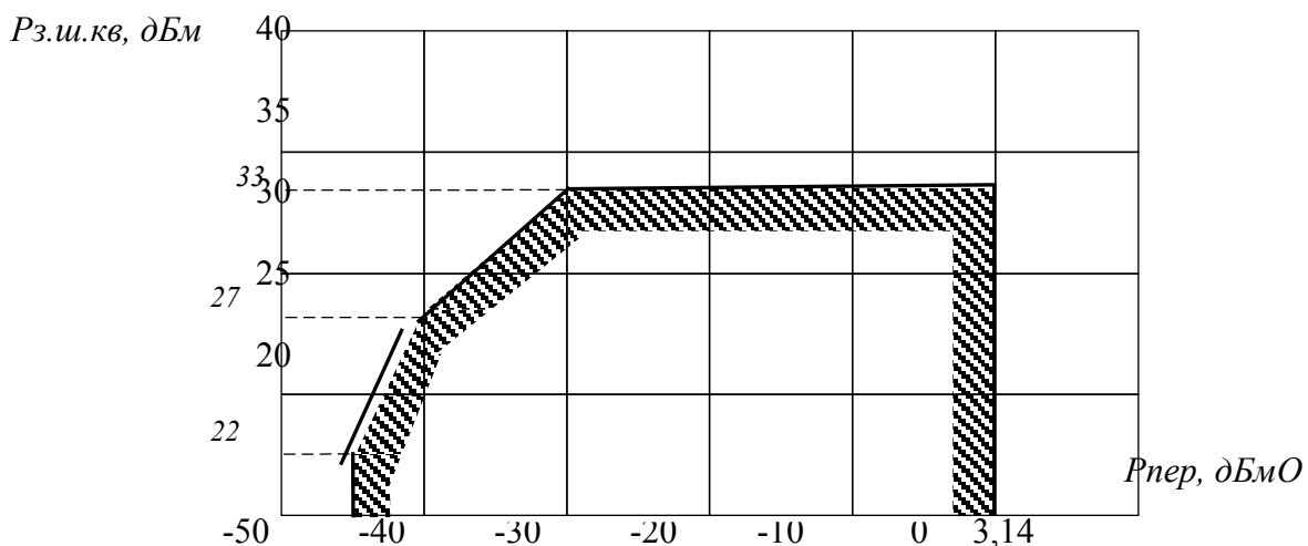
Рис. 2.8 – Шаблон защищенности от шумов квантования в канале ТЧ при измерении гармоническим сигналом =1010Гц
