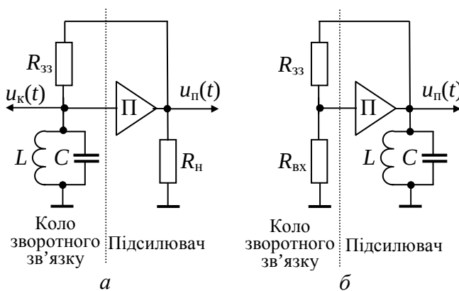
Рисунок 2 – LC -автогенератори з операційними підсилювачами
