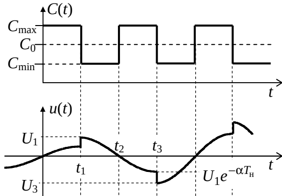
Рисунок 3 – Процеси, пов'язані з параметричною ємністю
