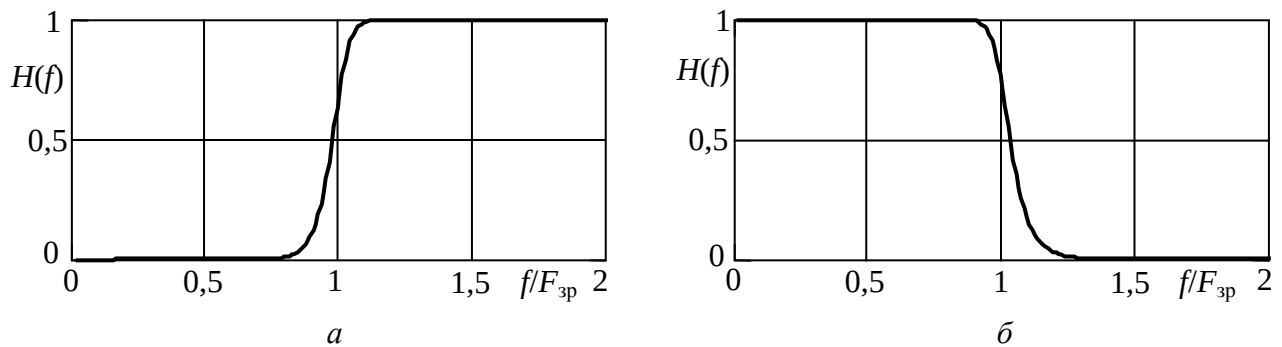
Рисунок 4 – АЧХ фільтрів: а – ФВЧ; б – ФНЧ
