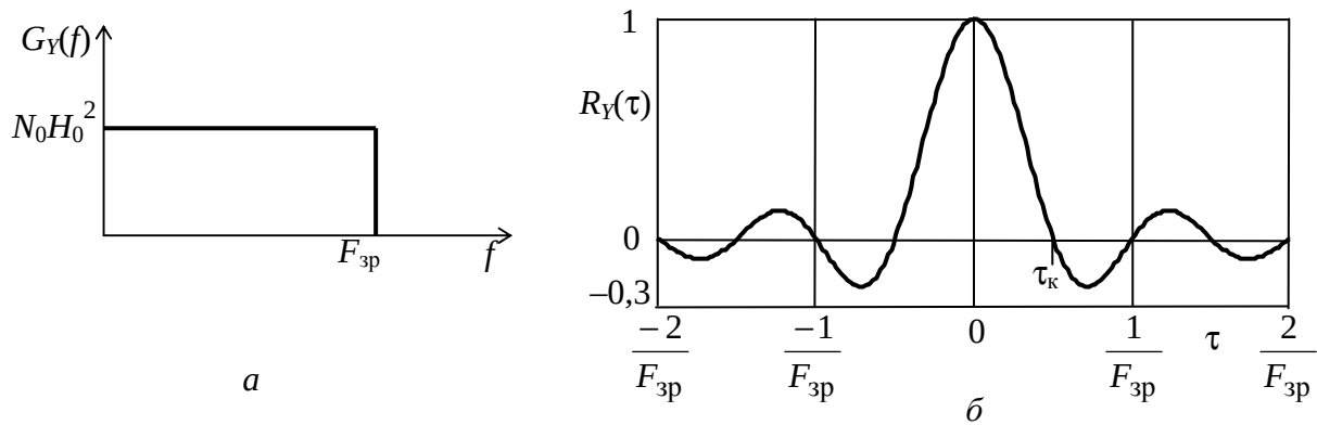
Рисунок 1 – Характеристики процесу Y(t) при фільтрації ФНЧ: a – СГП; б – КФ
