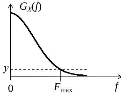
Рисунок 3 – Визначення ширини спектра
