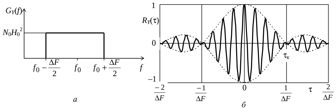
Рисунок 2 – Характеристики Y(t) при фільтрації смуговим фільтром: a – СГП; b – КФ
