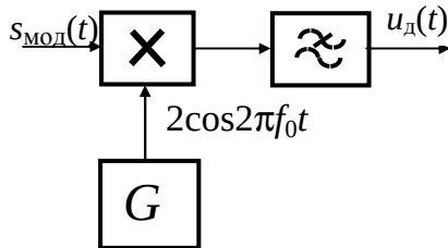
Рисунок 1 – Схема синхронного детектора
