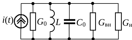
Рисунок 4 – Еквівалентна схема одноконтурного підсилювача
