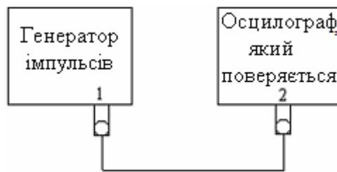
Рисунок А.2 – Схема визначення ширини лінії променя у вертикальному напрямку: 1 – вихід основних імпульсів; 2 – вихід підсилювача
