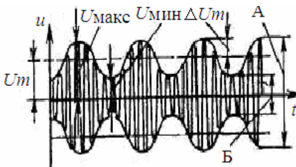
Рисунок 1.3 – Амплитудно-модулированные колебания
