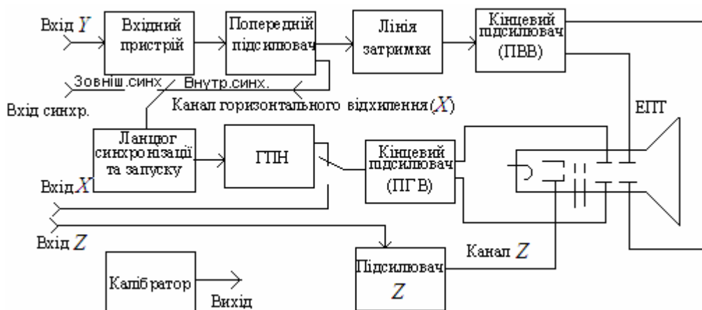
Рисунок 2.1 – Структурна схема універсального осцилографа
