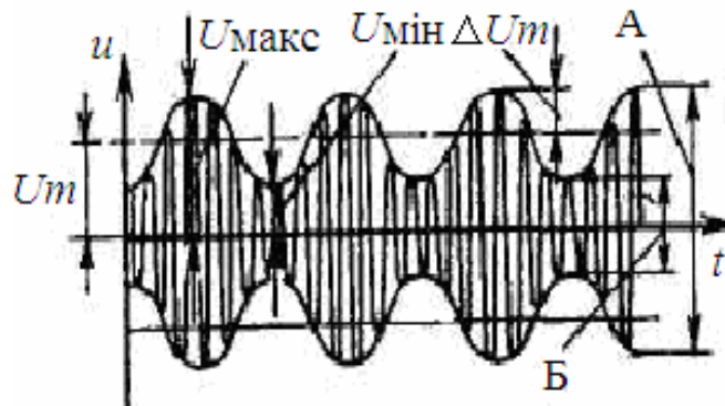
Рисунок 1.3 – Амплітудно-модульоване коливання
