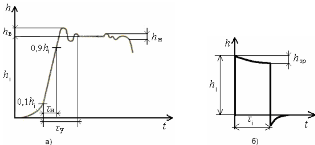
Рисунок 1.1 – Параметри ПХ (а) і визначення спаду вершини (б)
