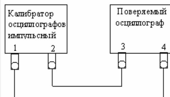
Рисунок А.8 – Схема измерения коэффициент развертки при применении калибратора осциллографов импульсного
