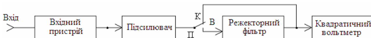
Рисунок 2.3 – Структурна схема вимірювача нелінійних спотворень
